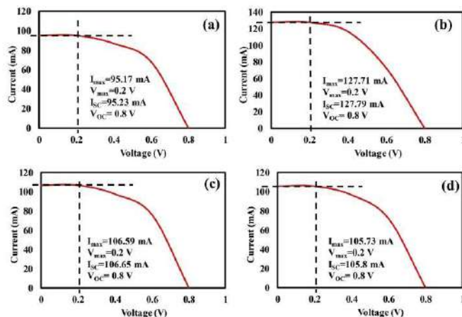
Fig. 12. PV response of (a) 0.5 wt%, (b) 1 wt%, (c) 1.5 wt% and (d) 2 wt% \text{TiO}_2 nanoparticles loaded PANI-graphene composites.
