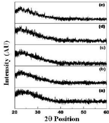
Figure 2 XRD of 60\text{V}_2\text{O}_5-5\text{P}_2\text{O}_5-(35-x)\text{B}_2\text{O}_3-x\text{Na}_2\text{O}_2 for (a) 5 mol %, (b) 10 mol %, (c) 15 mol %, (d) 20 mol % and (e) 25 mol % of \text{Na}_2\text{O}_2 .
